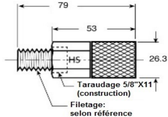
Coupleur 1" Fas Tie
