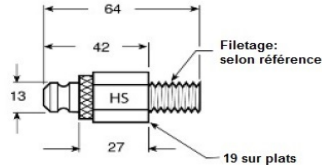
Embout 1" Fas Tie
