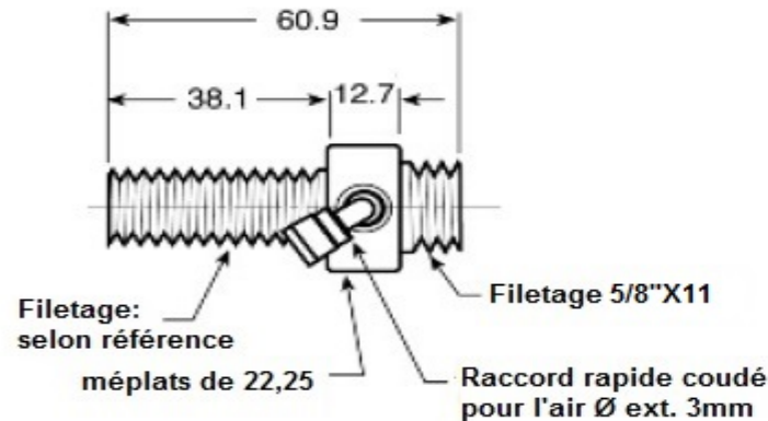
Adaptateur 1" Fas Tie
